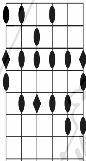
2. Dórica b2
