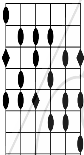
4. Lidia b7
