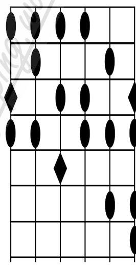
7. Alterada (superlocría)
