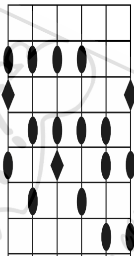
3. Lidia #5
