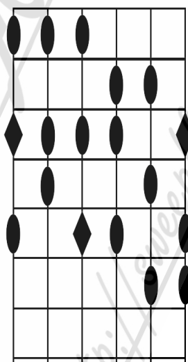
6. Eólica b5
