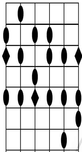
1. menor Melódica
